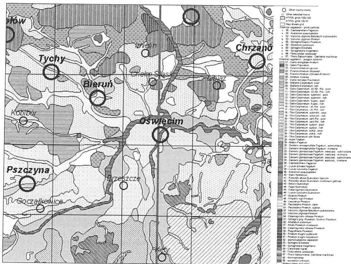
Rys. 7 Potencjalna roślinność naturalna.
