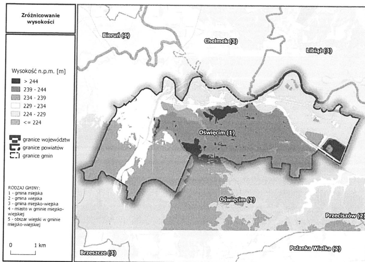
Rys. 3 Zróżnicowanie wysokości terenu n.p.m. [m].
