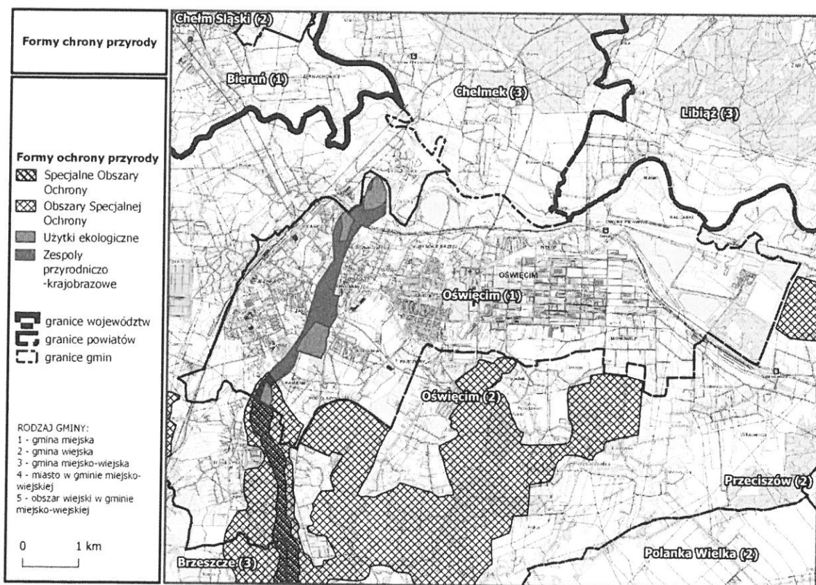
Rys. 9 Formy ochrony przyrody.
